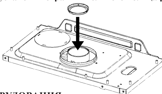
Схема установки ограничительного кольца рис.13
